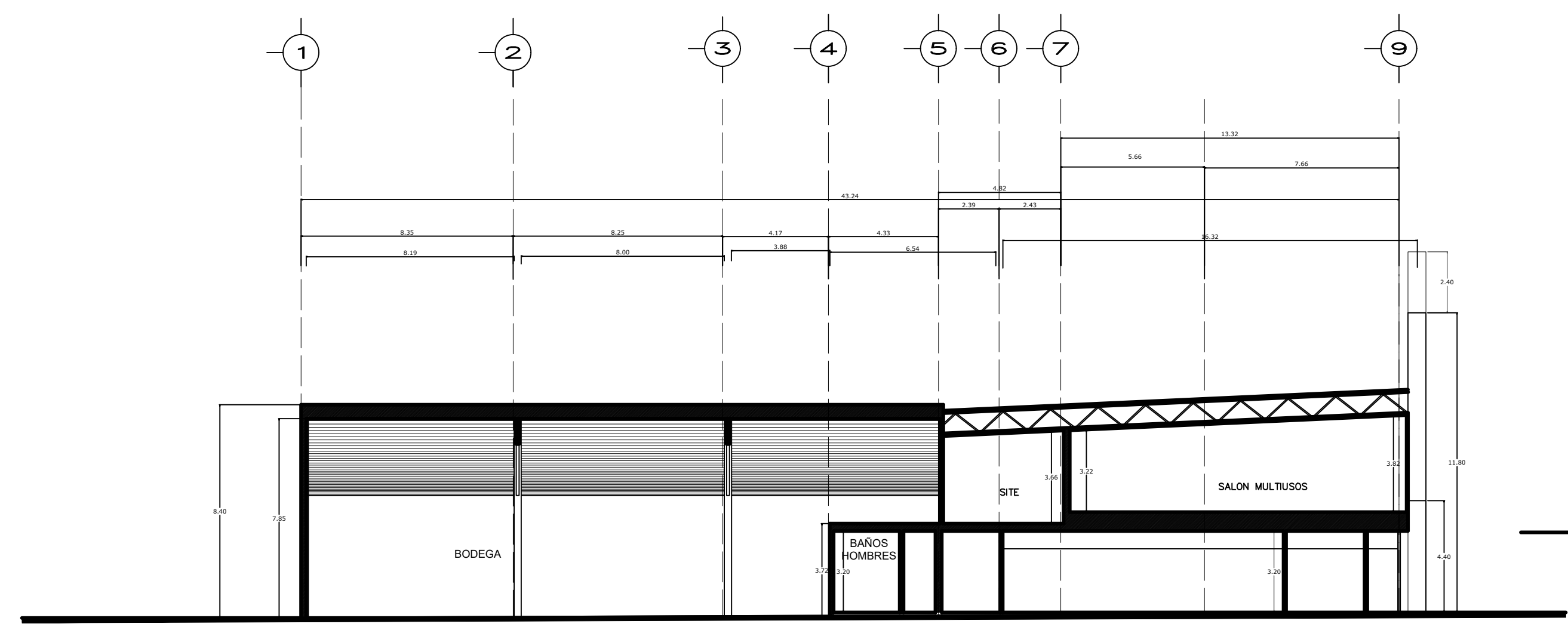
SECCION X-X'
