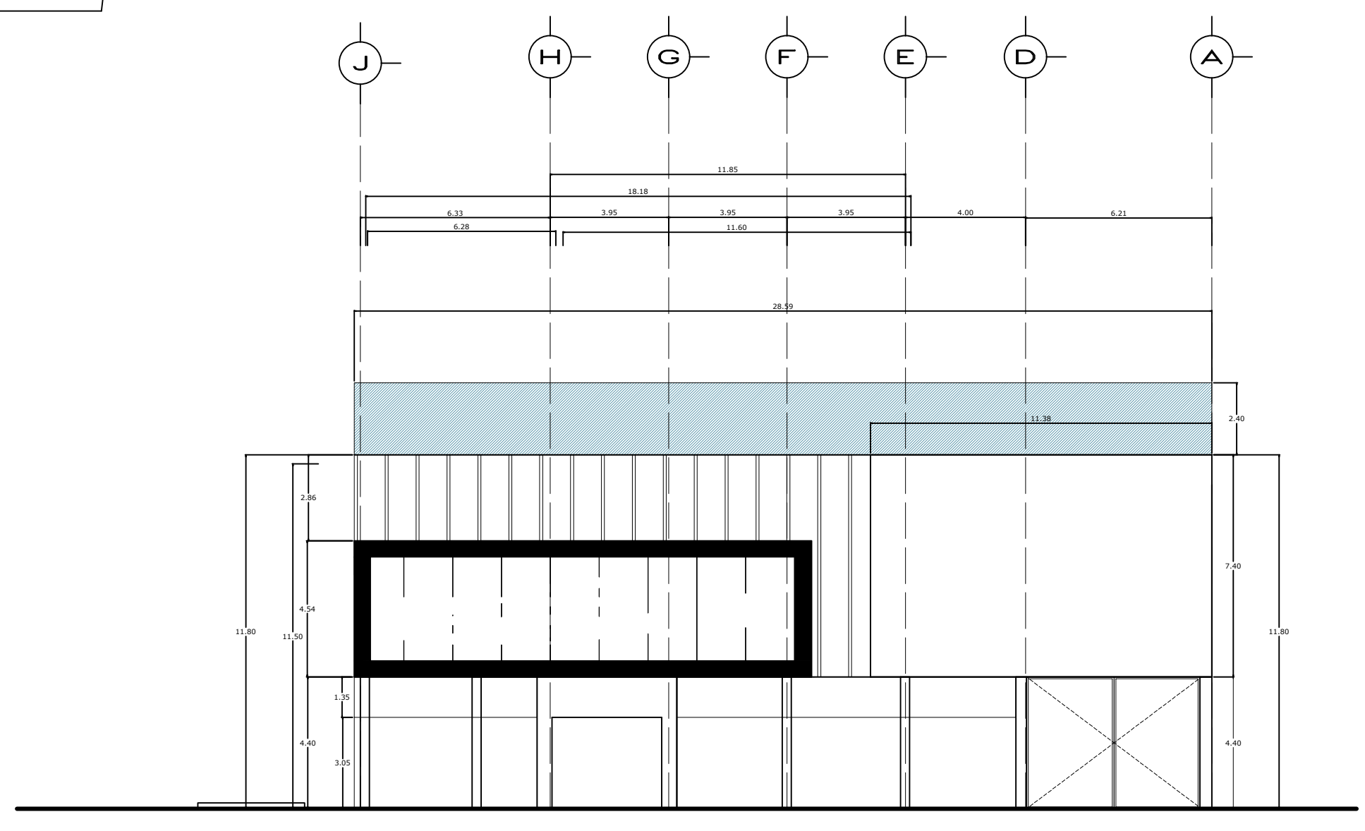
ALZADO FRONTAL
