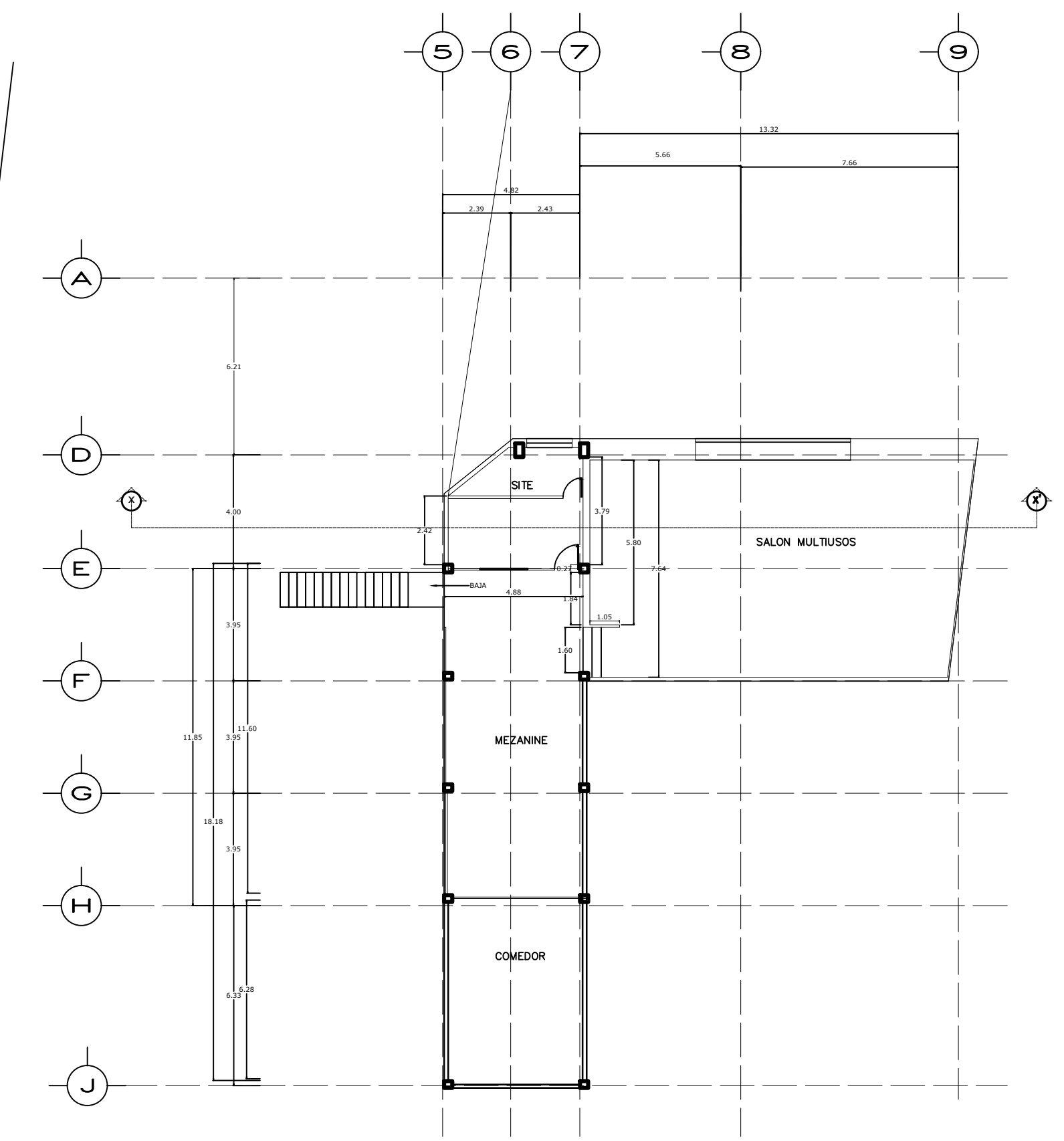
PLANTA ALTA
