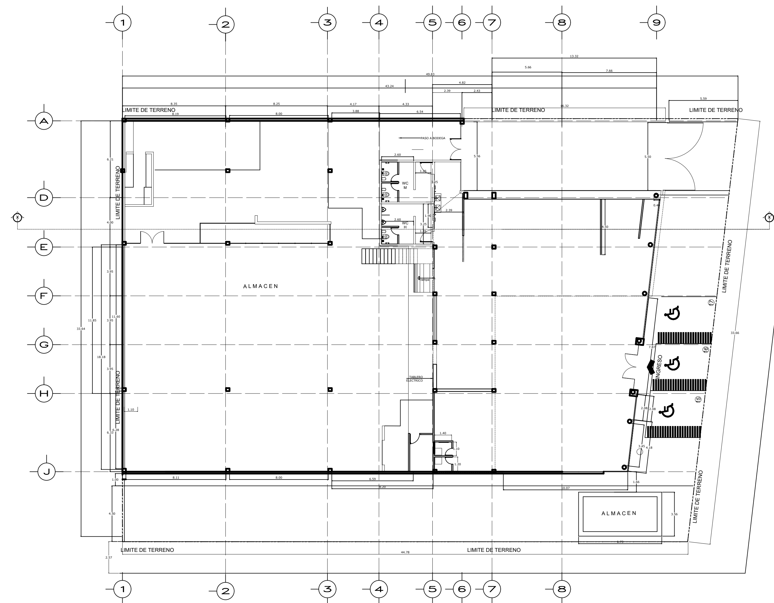
PLANTA BAJA
